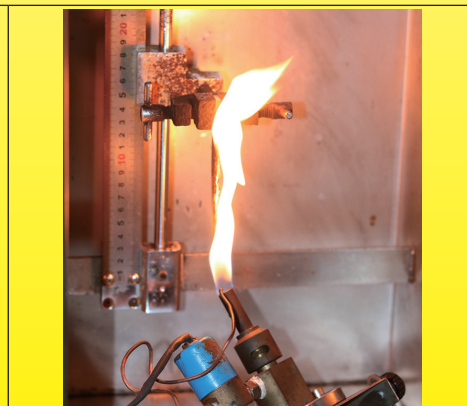
Образец во время испытания на UL94VO
